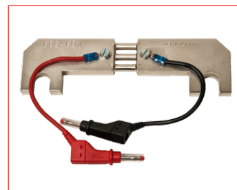
校准负载， 600 A/60mV (BB-90020)
