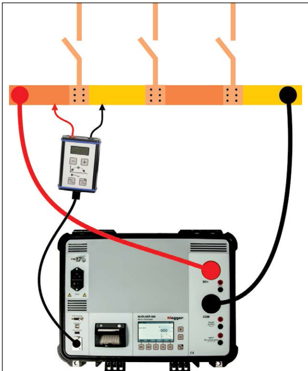
使用远程控制可以测量被测母线的每个部分内的每个触点元件的电压降（电压）。
