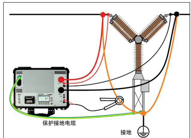
测试过程中试品的两端都可接地，提高了测试的安全性。
